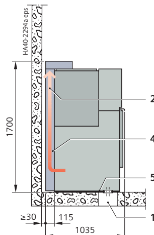
Anlagenaufstellung mit Druckentlastungskanal (Option)
