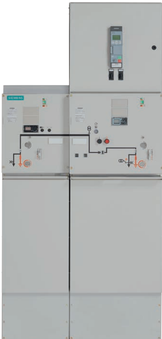
Ringkabelfeld und Leistungsschalterfeld als Einzelfelder
