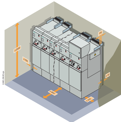
Anlagenaufstellung mit Druckentlastungskanal und optionalem Absorber
