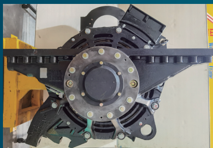
HXD1B型牵引电机 驱动端 Driving Side
