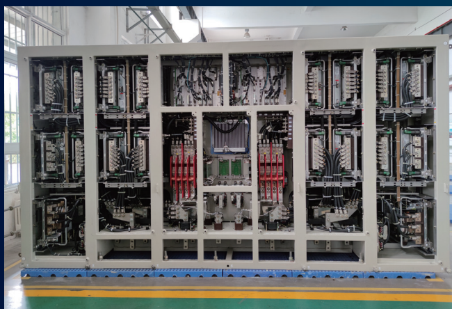
HXD1型电力机车主变流器 HXD1 Locomotive Main Inverter
