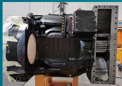
HXD1B型牵引电机 抱轴侧 Nose-Suspension Side
