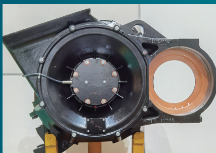
HXD1B型牵引电机 非驱动端 Non-Driving Side
