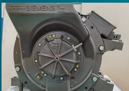
HXD1型牵引电机 非驱动端 Non-Driving Side
