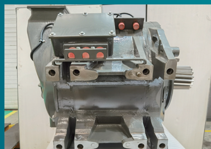
HXD1型牵引电机 抱轴侧 Nose-Suspension Side
