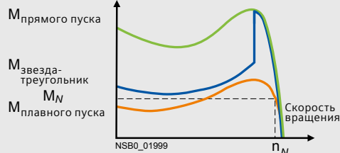
Момент двигателя
