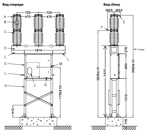
Габаритные чертежи ЗАФ
