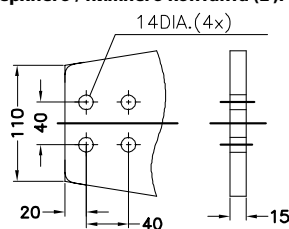
Алюминиевая контактная площадка верхнего / нижнего контакта (E, F)
