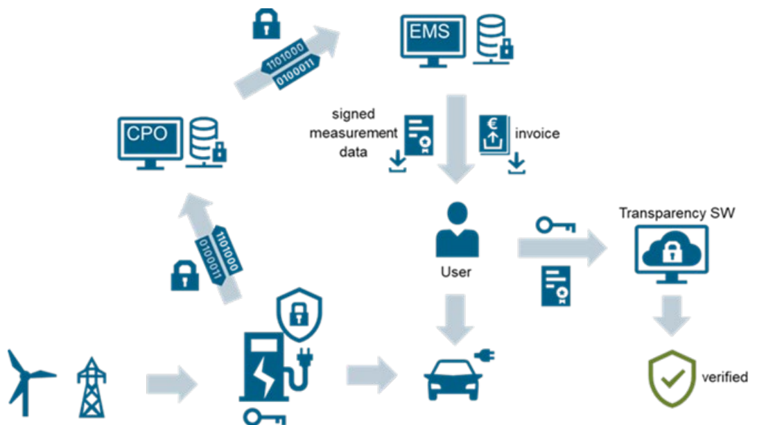
Bild 4-6 Integritätsprüfung des Ladevorgangs
