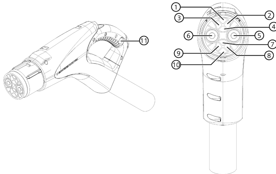
Bild 3-6 CHAdEMO-Stecker
