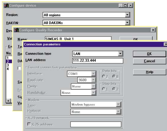
Fig. 13/76 Connection parameters
