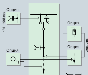
Тип R1 500 мм в ширину
