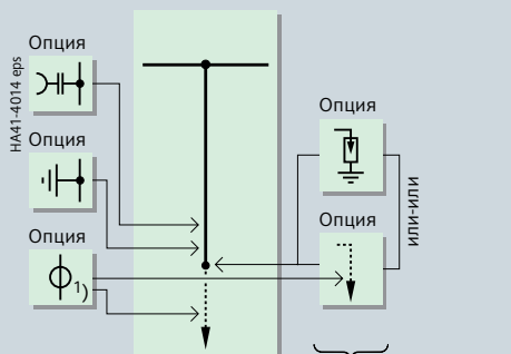
Тип К1 500 мм в ширину или: Исполнение с соединительными настройками
