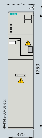
Тип Н, для передачи налево (без трансформатора)
