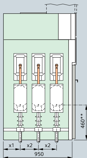
Измерительная ячейка, тип М(-ВК) (для присоединения сборных шин)
