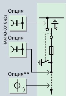
Тип T 375 мм в ширину
