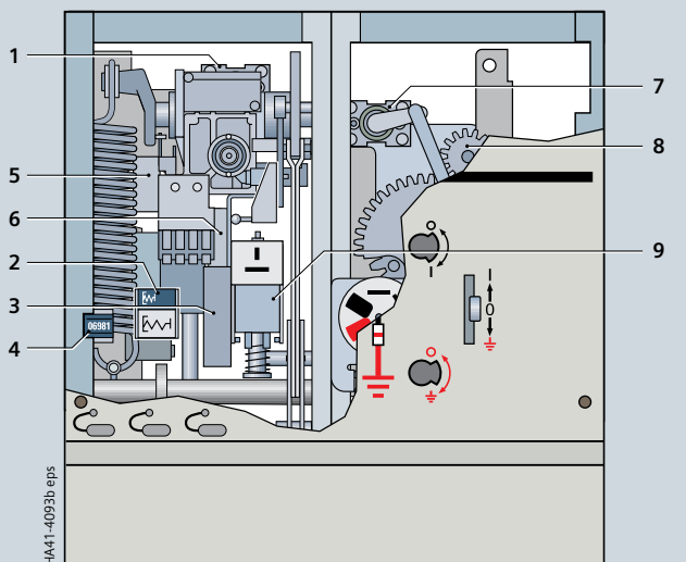
Вакуумный силовой выключатель, тип CB-f AR *)
