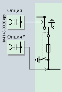
Тип T(T) 375 мм в ширину
