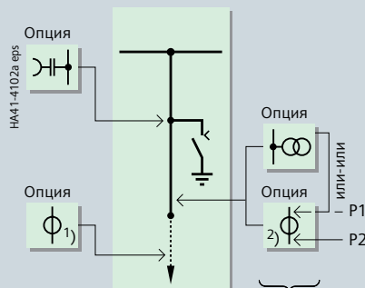
Тип К1 500 мм в ширину или: Исполнение с трансформаторами
