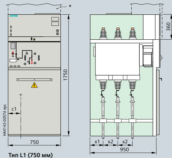
Тип L1 (750 мм)
