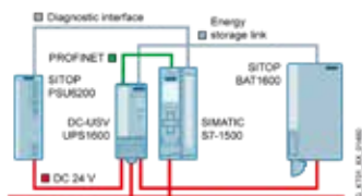
Módulo UPS
