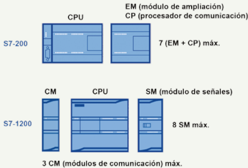
E/S integradas de la CPU y E/S de la SB (Signal Board)
