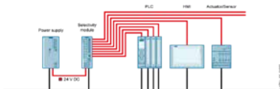
Módulo de selectividad
