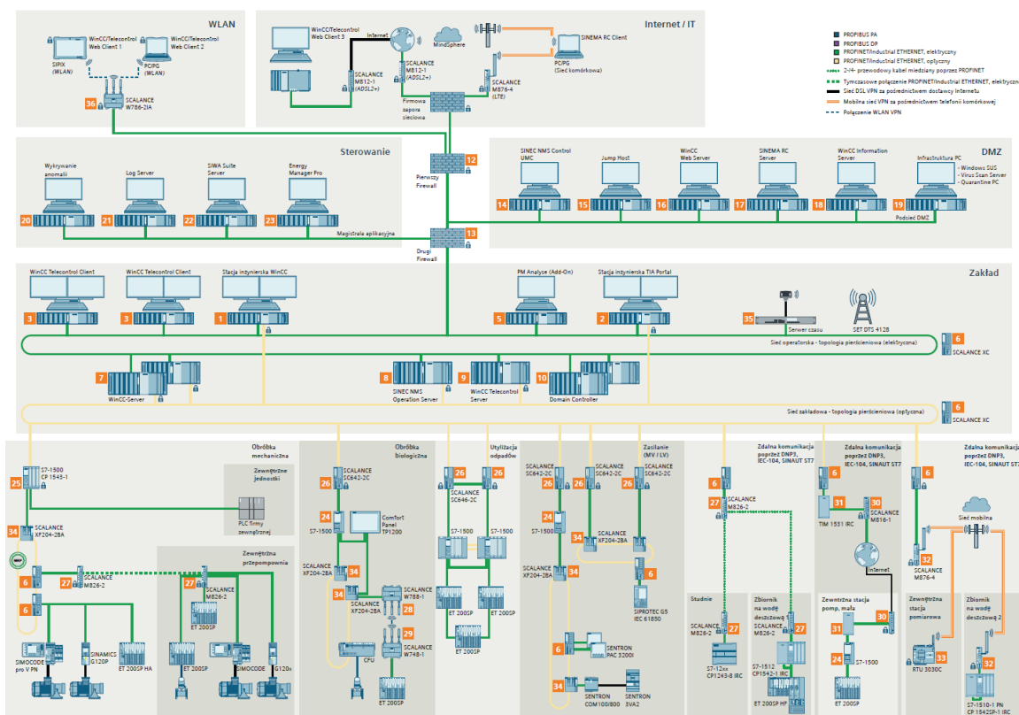
Ilustracja 6: Architektura systemu oparta na WinCC V7
