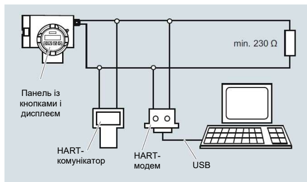
Комунікація HART
