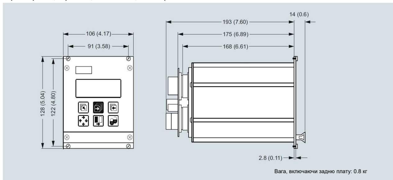
Розміри в мм (дюйм)
