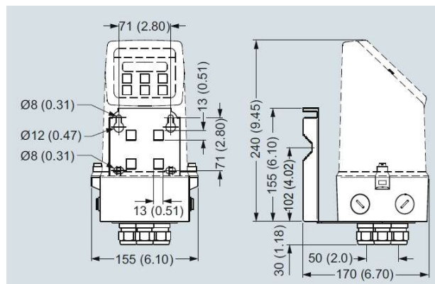
Перетворювач, монтаж на стіні, розміри в мм (дюйм)
