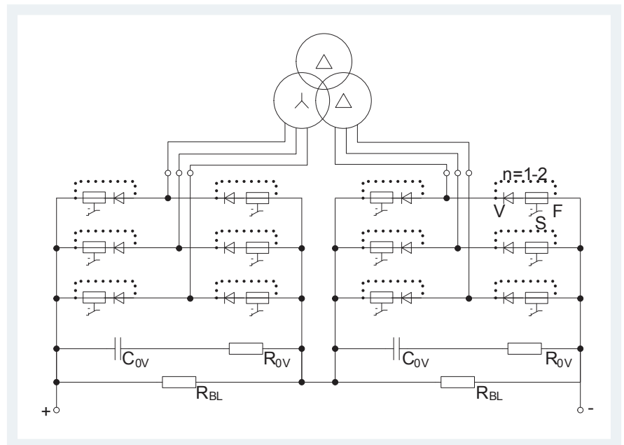
Reihenschaltung 6-pulsige und 12-pulsige Ausführung, DC 3000 V Typen: B6U2S 3000P1, B6U2S 3000P2 (Option: DC 600 / 750 V und DC 1.500 V)
