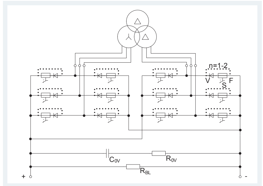
Parallelschaltung 6-pulsige und 12-pulsige Ausführung, DC 600 / 750 V und DC 1.500 V Typen: B6U2P 750P1, B6U2P 1500P1, B6U2P 750P2, B6U2P 1500P2
