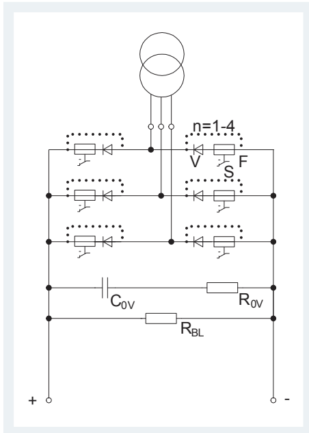
6-pulsige Ausführung, DC 600 / 750 V und DC 1.500 V Typen: B6U 750P1, B6U 1500P1, B6U 750P2, B6U 1500P2, B6U 750P3, B6U 1500P3, B6U 750P4, B6U 1500P4
