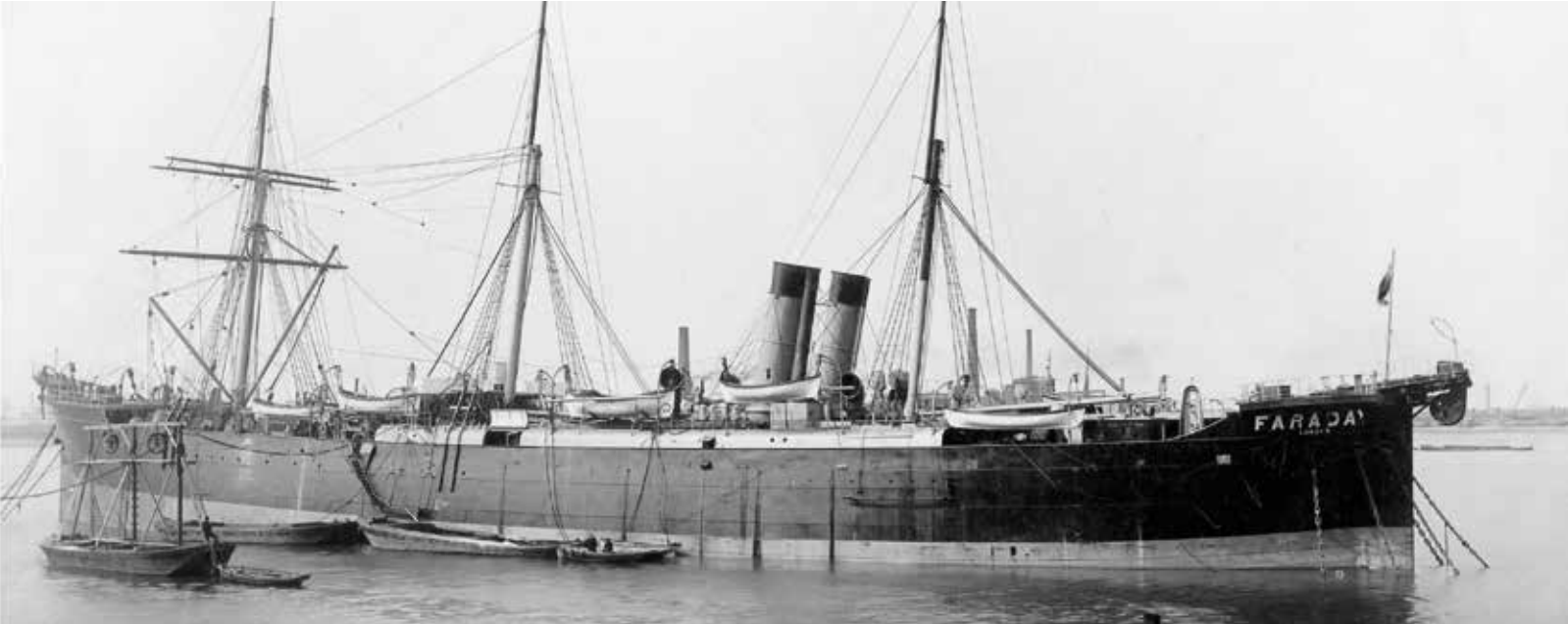
A mélytengeri kábelfektetésre kialakított hajó, a Faraday, 1874
