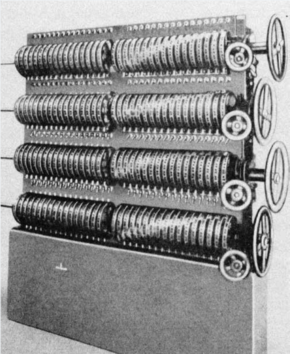
A Magyar Művelődés Háza színpadi világításának 128 karú új színpadi állítóműve
