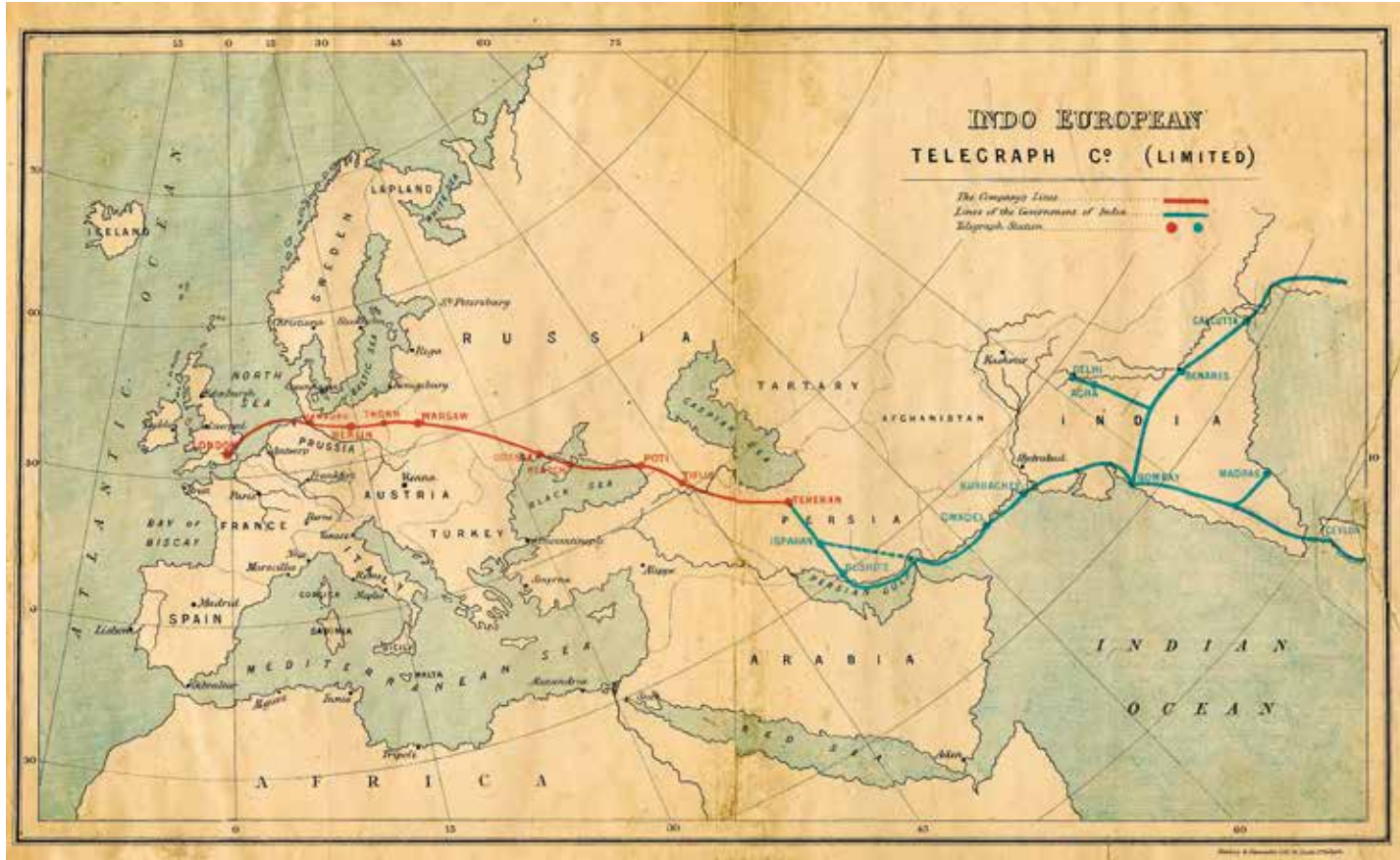
A Londontól Calcuttaig húzódó indoeurópai távírvonal, 1870 körül
