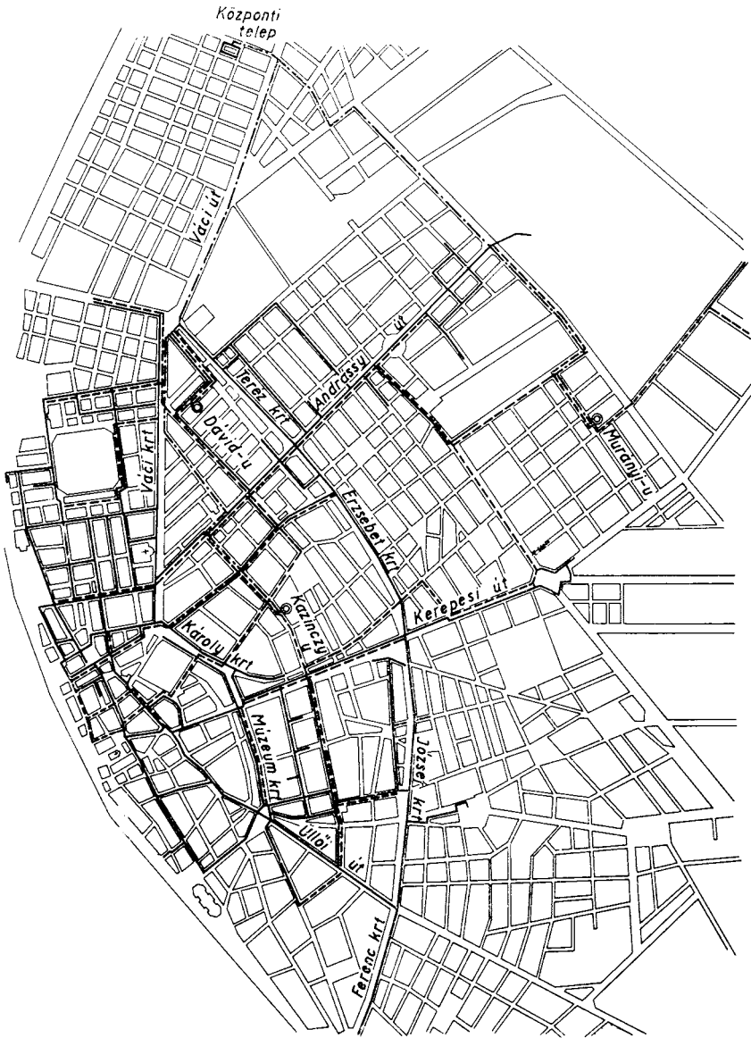
A budapesti egyenáramú hálózat 1895-ben
