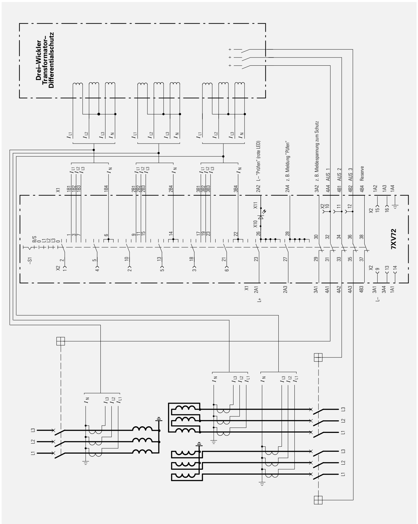
Bild 5 Anschlußschaltplan für Prüfshalter 7XV7202-0CA00
