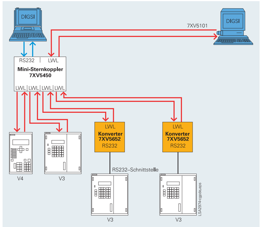
Abb. 13/58 Fernabfrage mit der RS232-Schnittstelle
