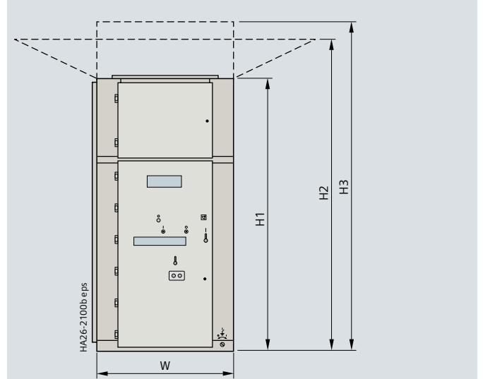
Önden görünüm
