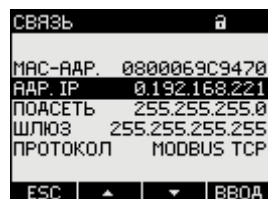
Изображение 9-10 Настройка устройства «СВЯЗЬ»
