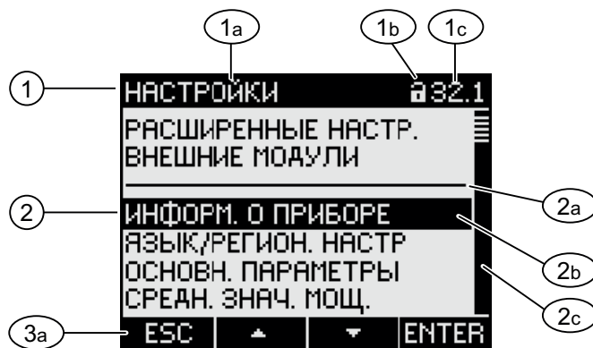
Изображение 8-10 Индикация «НАСТРОЙКИ»
