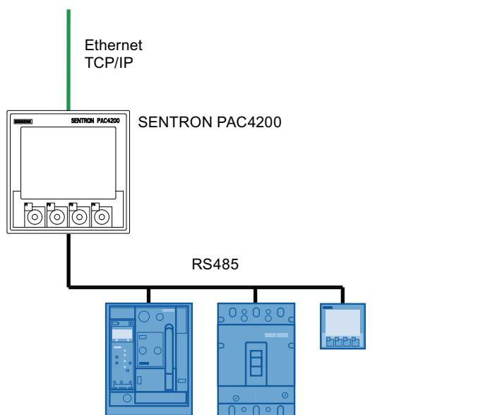
Изображение 3-18 SETRON PAC4200 в качестве шлюза
