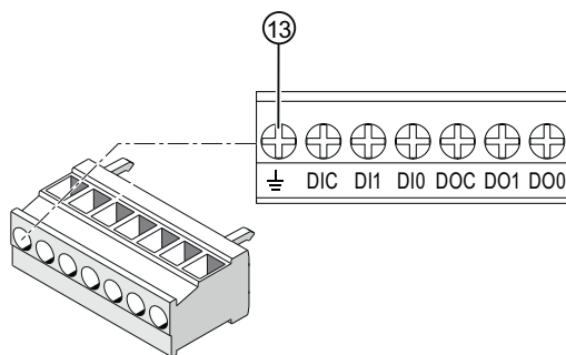
(13) Клемма функционального заземления
