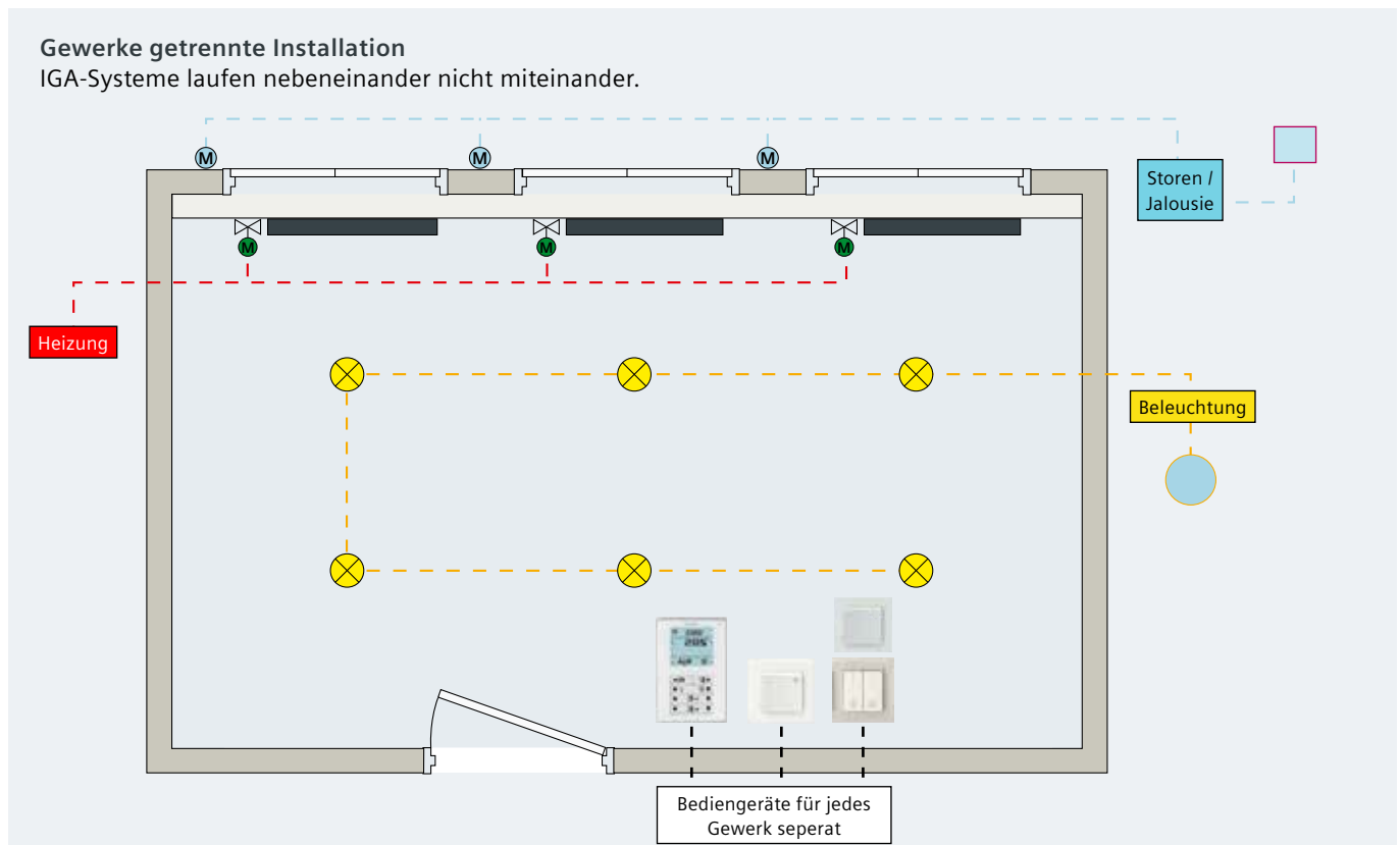
Abb. 2: Gewerkegetrennte Installation
