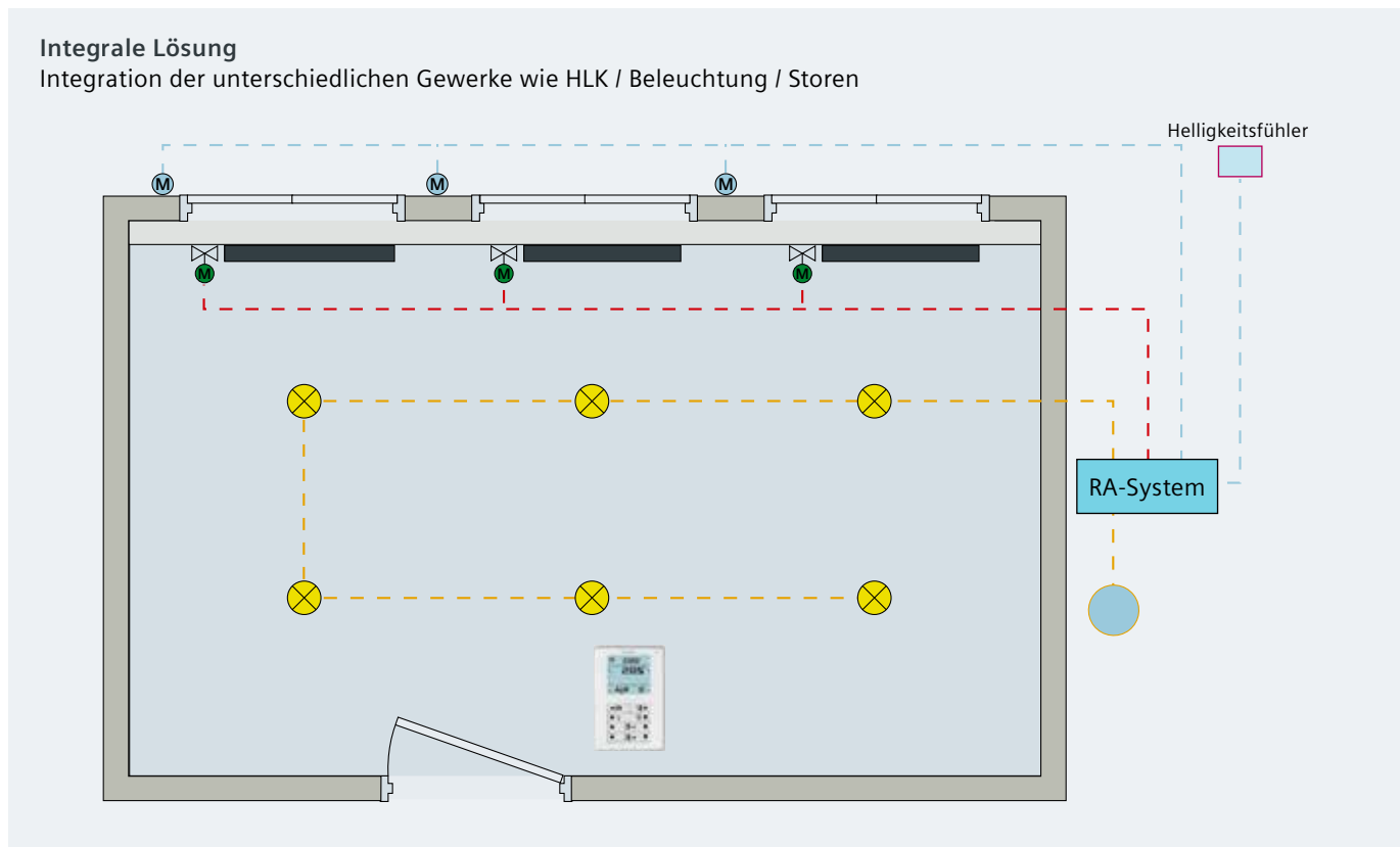
Abb. 3: Gewerkeintegrierte Installation
