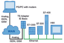
Teleservis Adaptörü
