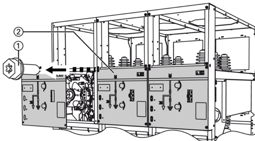
Рисунок 75: Демонтировать крышки панелей управления
