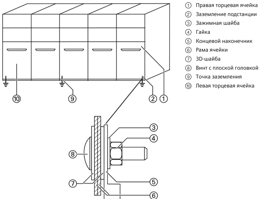
Рисунок 91: Рама распределительного устройства с точкой заземления (резьбовое соединение M12)
