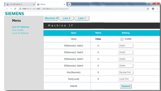
Parameters set from web browser
