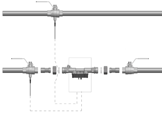
6: Példa érzékelő fogadó golyócsapos beépítéssel (ajánlott DN25 méretig)
