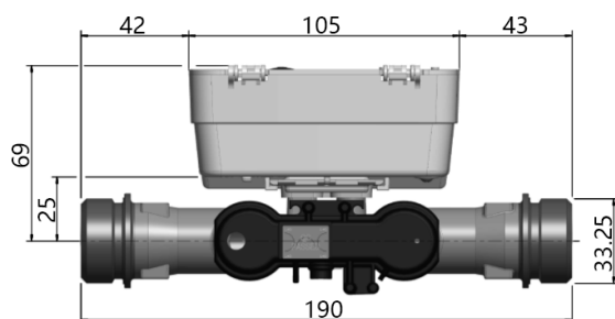
5: Méretek áttekintése a 190 mm beépítési hosszú mérőknél (menetes)
