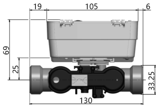
4: Méretek áttekintése a 130 mm beépítési hosszú mérőknél (menetes)
