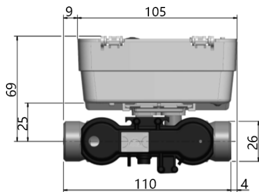
3: Méretek áttekintése a 110 mm beépítési hosszú mérőknél (menetes)
