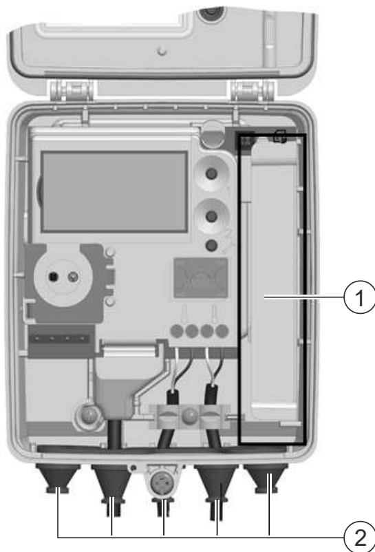
1 Kommunikációs modul 2 Bekötő csomok
