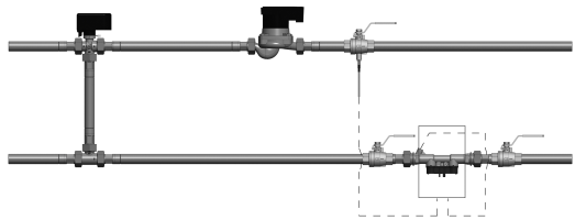
7: Beépítési példa keverő alkalmazás mellett; Hőmérsékletérzékelő beépítési helye
