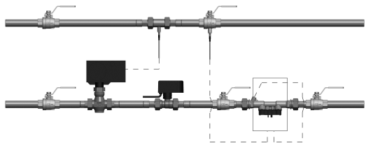
8: Beépítési példa fojtó szelepes körnél (előremenő érzékelő az előremenőben a szabályzó szelep / nyomáskülönbség szabályzó előtt)
