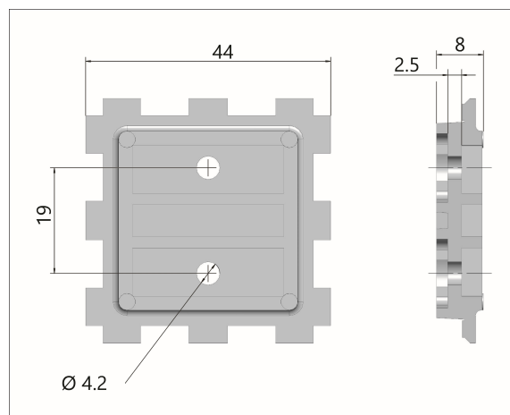
2: Az adapter lap felülnézete és oldalnézete
