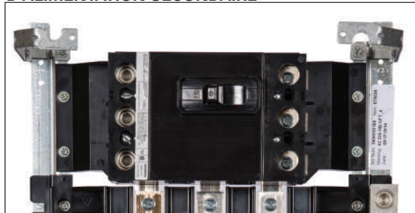
COSSES PRINCIPALES ou COSSES DE PASSAGE
