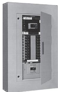
Panneau d'éclairage à disjoncteurs de type P1
