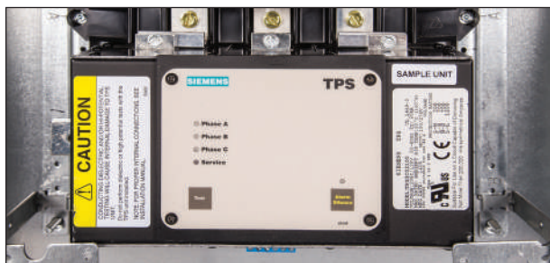
PARASURTENSEUR INTÉGRAL SUR LA BARRE OMNIBUS
