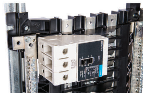
Exemple de disjoncteur principal xGB alimenté par l'arrière
