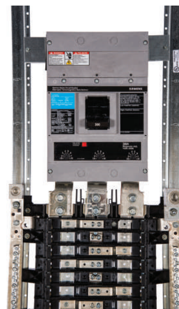
Disjoncteur principal de 300 A installé.
