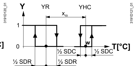
Režim chlazení
