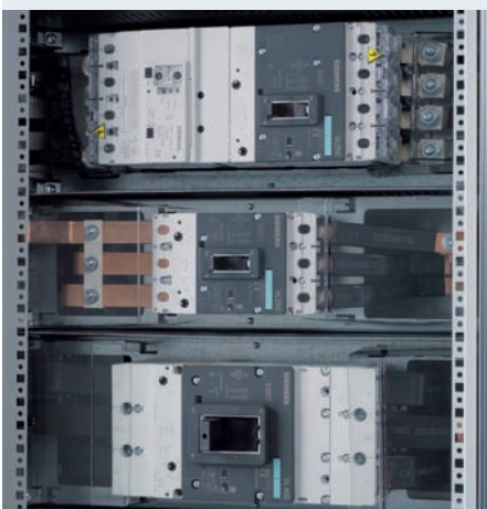
Kit di montaggio per interruttori automatici scatolati SENTRON 3VL
