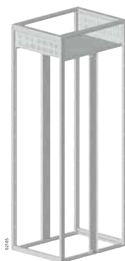
Sistema di sbarre principali in posizione standard superiore frontale e posteriore P = 800 mm.
