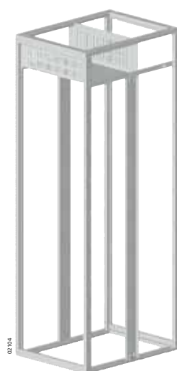
Sistema di sbarre principali in posizione standard superiore frontale o posteriore P = 800 mm.
