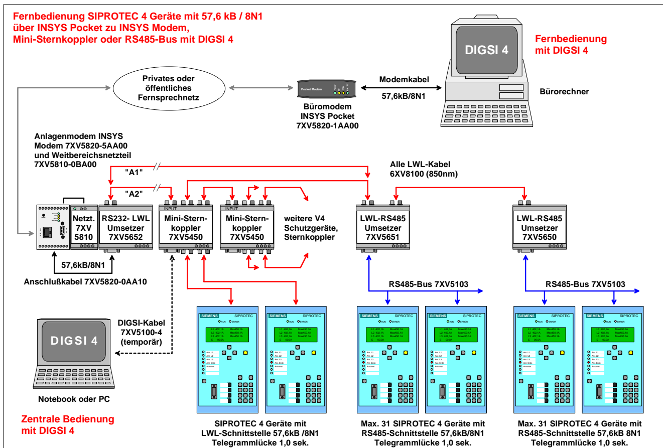
Bild 1: Die Hardwarestruktur einer zentralen, bzw. Fernbedienung von SIPROTEC 4 Schutzgeräten.
