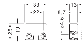
3SX3 261 spacer
