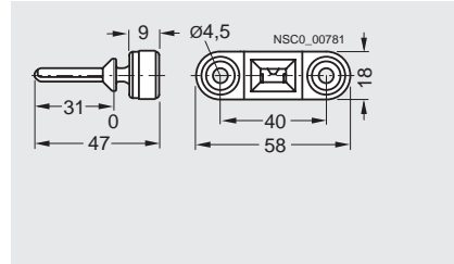
3SE5 000-0AV05 universal radius actuator
