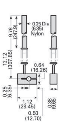
Nylon Spring Rod Actuator 3SX03-KL556
