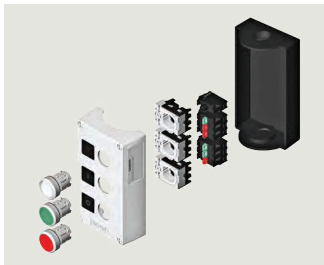
I/O Link Enclosure
