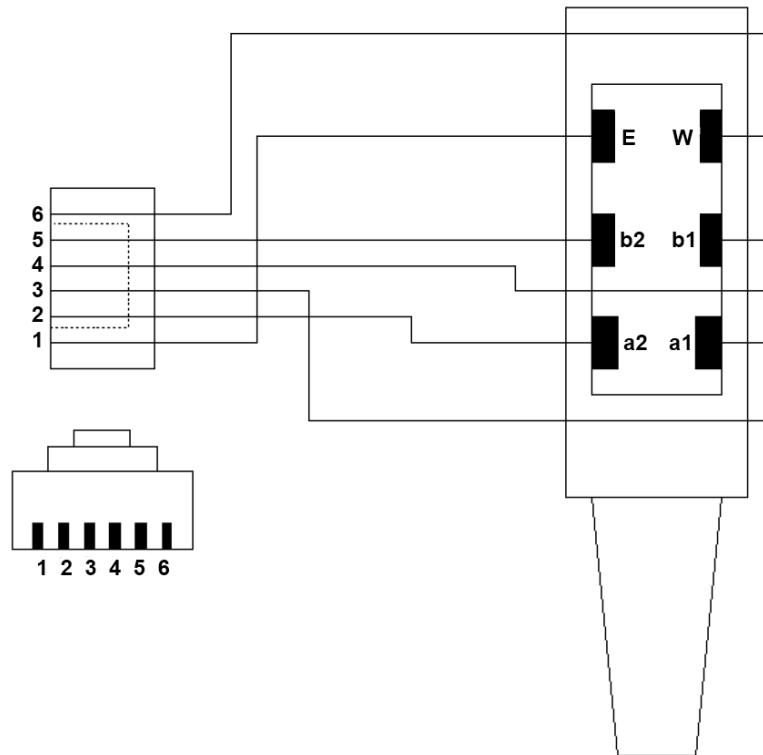
Abbildung 4: RJ12-Stecker verbunden mit TAE-Stecker
