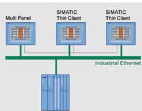
Thin Client'tan Sm@rtServer Operatör Panele bağlantı
