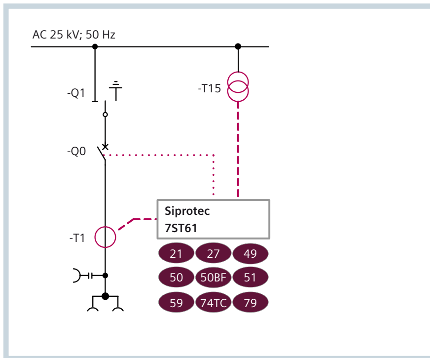
Typische Konfiguration eines AC-Abgangsfeldes mit digitalem Oberleitungsschutzgerät (enthält optionale Funktionen)
