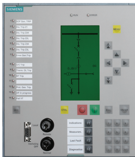
Bedienfelder Schutzgerät Siprotec 7ST61 (oben) und kombiniertes Schutz- / Steuergerät Siprotec 7ST63 (Ausschnitt, unten)
