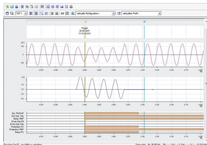
Störfalldarstellung mit der Diagnosesoftware Sigrá 4
