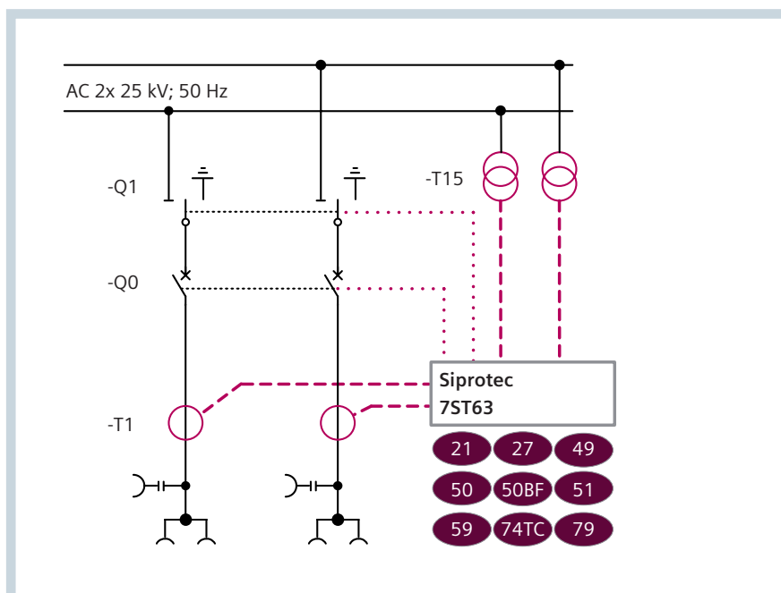
Typische Konfiguration eines AC-Abgangsfeldes im Autotransformator-System mit digitalem Oberleitungsschutz- und -steuergerät (enthält optionale Funktionen)
