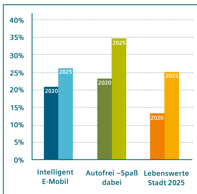
Abbildung 19: Einsparungen PM10 [%], tank to wheel (lokal in der Stadt)
