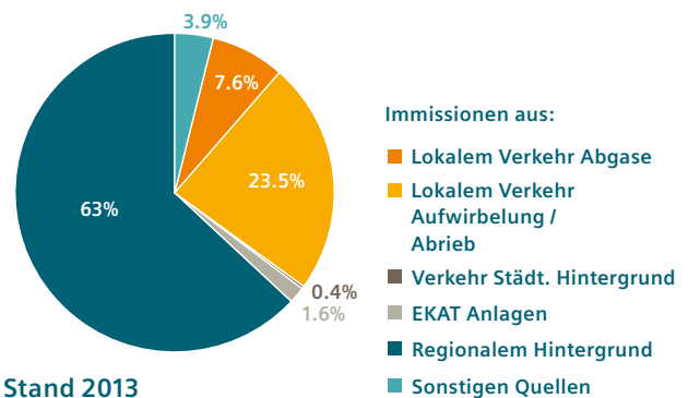
Abbildung 7: Beiträge unterschiedlicher Quellen zur Feinstaubbelastung (Beispiel 2013, Von-der-Tann-Straße) [RUS 2015]
