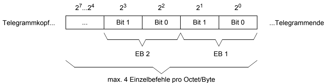
Bild 3-2 Datentyp Einzelbefehl
