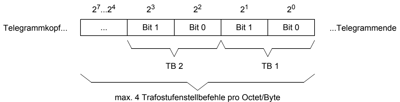
Bild 3-7 Datentyp Trafostufenstellbefehl
