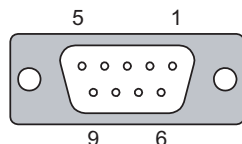
図 12-2 RS 422 インターフェースおよび RS 485 インターフェースのピンの割り付け
