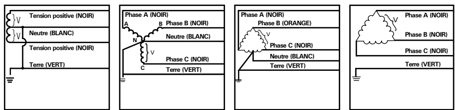
Figure 1 Partagé 2 tension positive, 1 neutre, 1 terre Figure 2 Étoile 3 tension positive, 1 neutre, 1 terre Figure 3 Triangle sous tension (B élevé) - 3 tension positive, (B élevé), 1 neutre, 1 terre Figure 4 Triangle et Étoile HRG 3 tension positive, 1 terre
