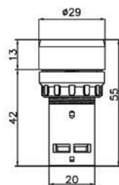
Botão monobloco
