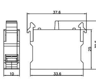
Sinaleiro monobloco (220V)
