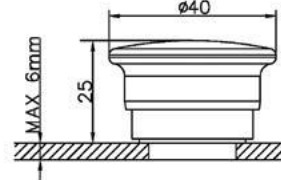
Botão de emergência ø 40mm mecanismo puxar para destravar
