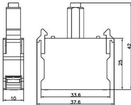
Botão monobloco
