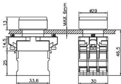
Botão de comando faceado com ou sem sinalização
