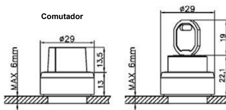
Comutador com chave
