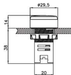
Sinaleiro monobloco
