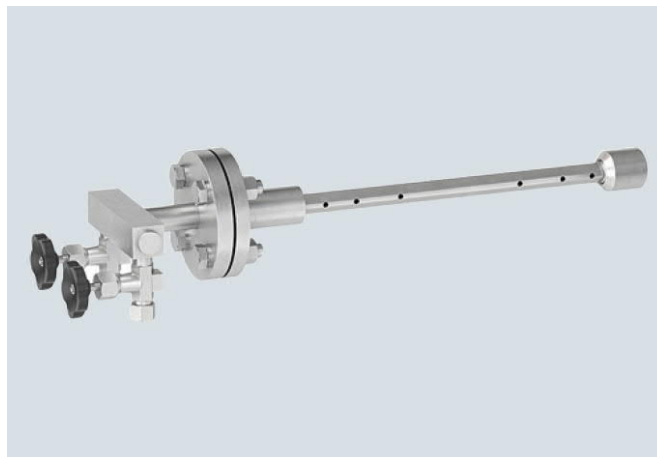
SITRANS FPS300 – роздільна конструкція
