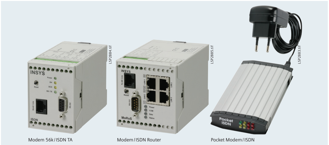
Abb. 13/79 Industrie-Modems
