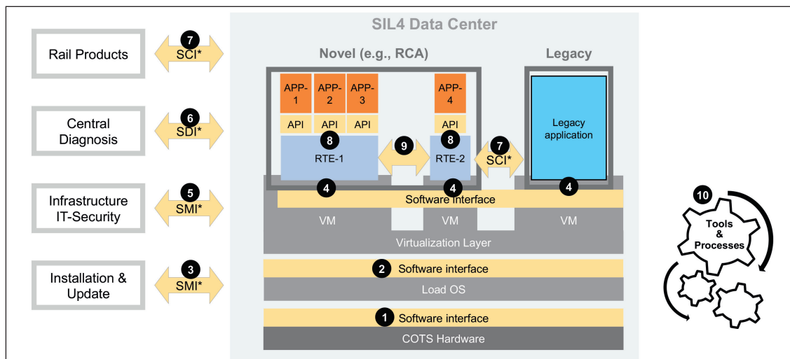
Bild 2: Schnittstellen zwischen den Komponenten eines SIL4 Data Centers
