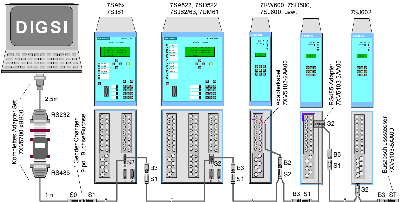
Bild 1: Zentrale Bedienung über RS485-Bus
