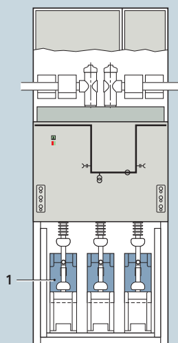
Установка трансформатора тока (базовая схема)
