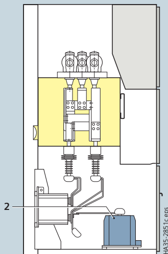
Установка трансформатора напряжения (базовая схема)
