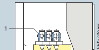
Ячейка со сборной шиной 1250 А
