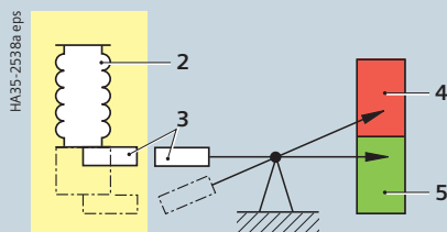
Панель управления (деталь) с красным / зеленым индикатором готовности к работе
