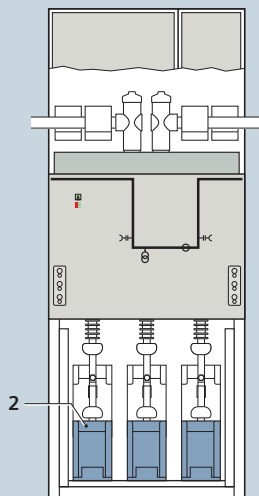
Установка трансформатора напряжения (базовая схема)
