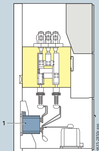
Установка трансформатора тока (базовая схема)
