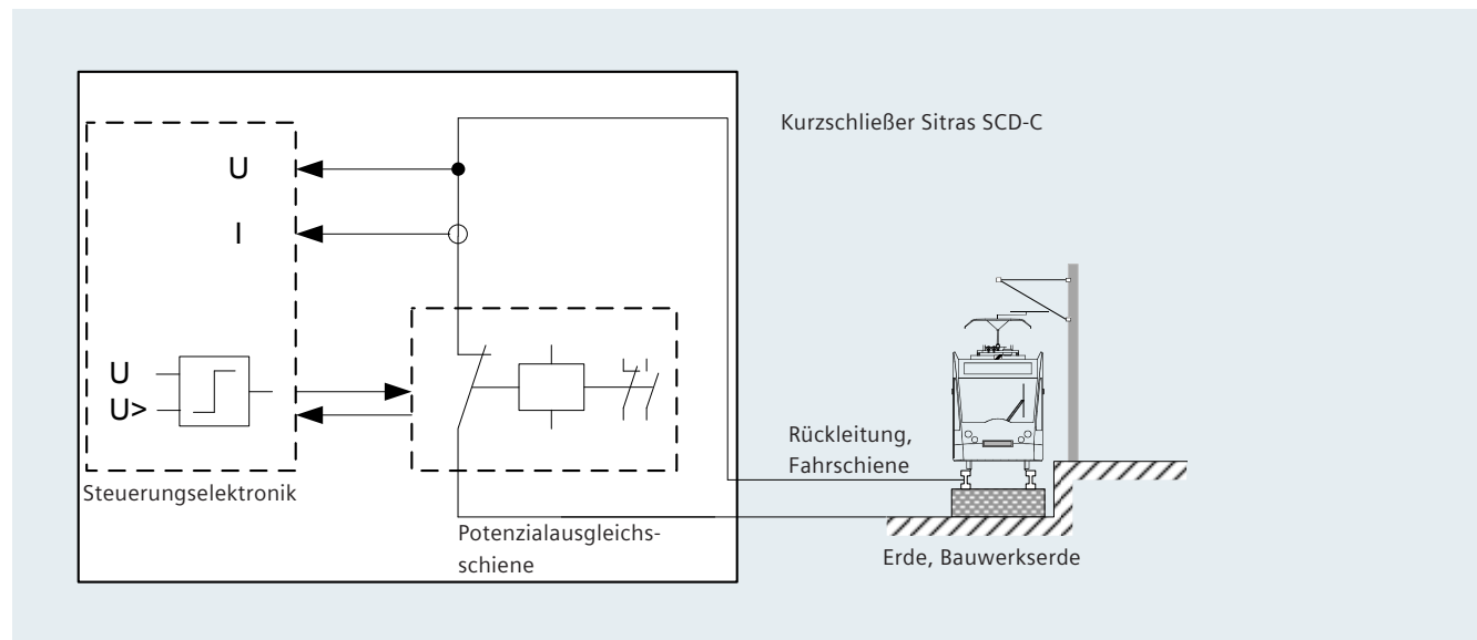
Prinzipschaltbild Sitras SCD-C
