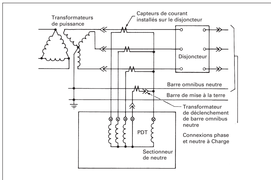
Figure 19. Schéma pour la protection contre les défauts à la terre d'un système à quatre fils, avec détection résiduelle
