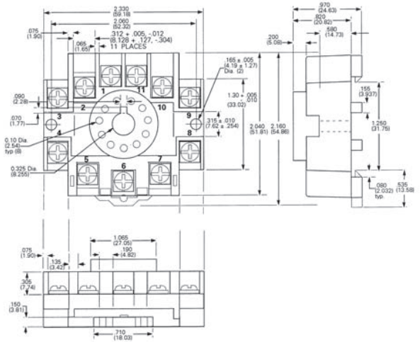
3TX7144-1E3
