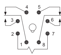
3TX7127 (DPDT)
