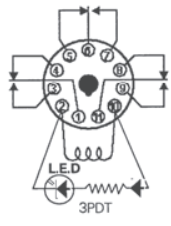
3TX7112
