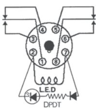
3TX7112
