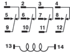
3TX7127
