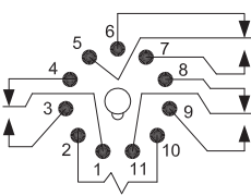
3TX7127 (3PDT)
