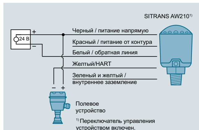
Внешний источник питания 24 В DC, подключение одного устройства
