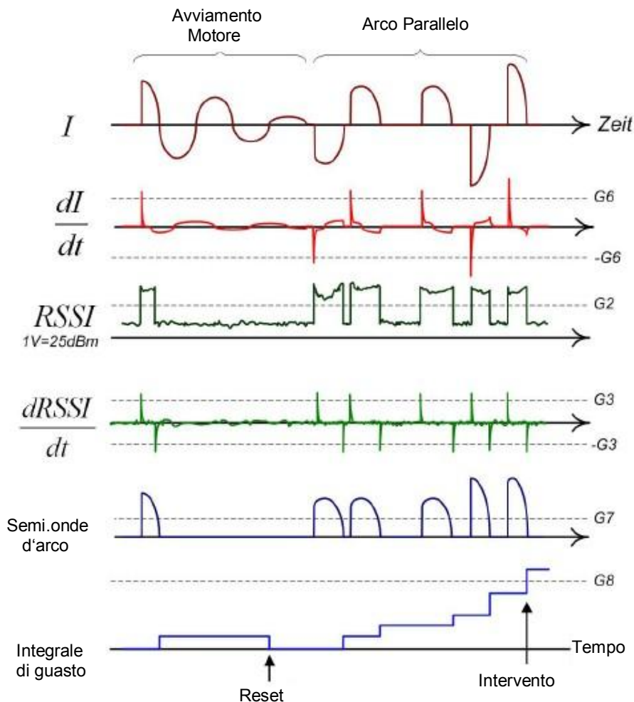
Figura 25: Processo di analisi del segnale per l'identificazione di guasti da arco parallelo
