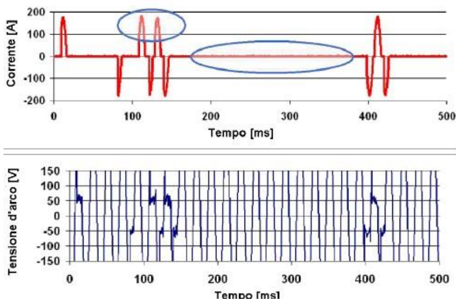
Figura 20: Curve di corrente e tensione per un guasto da arco in parallelo.
