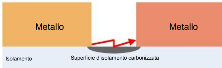
Figura 14: Arco elettrico su superficie isolante deteriorata.
