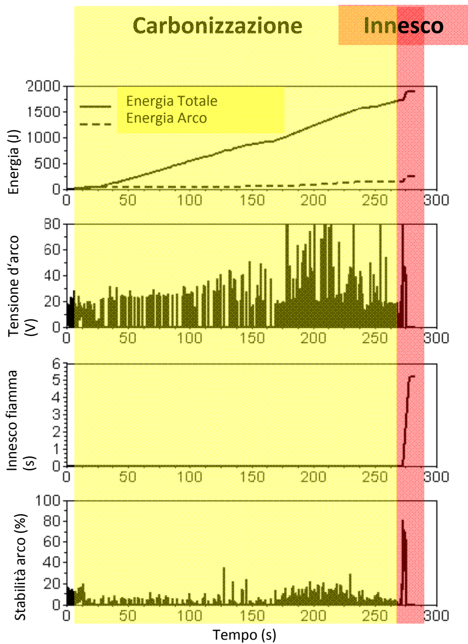
Figura 16: Simulazione di arco serie 2 A / 240 V
