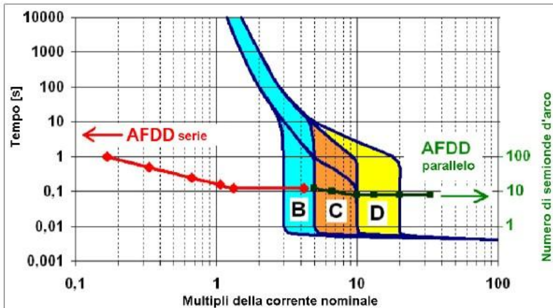
Figura 21: Protezione con interruttori automatici ( I_n=16A )
