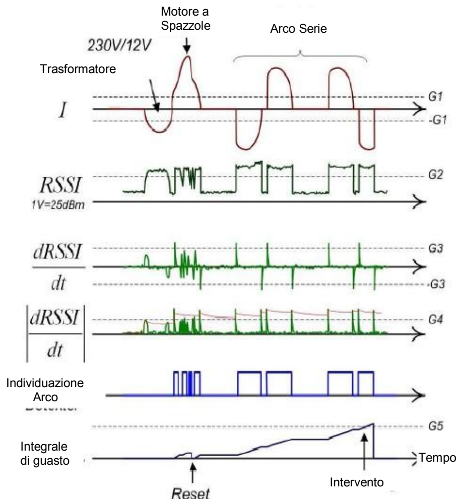
Figura 24: Processo di analisi del segnale per l'identificazione di guasti da arco serie
