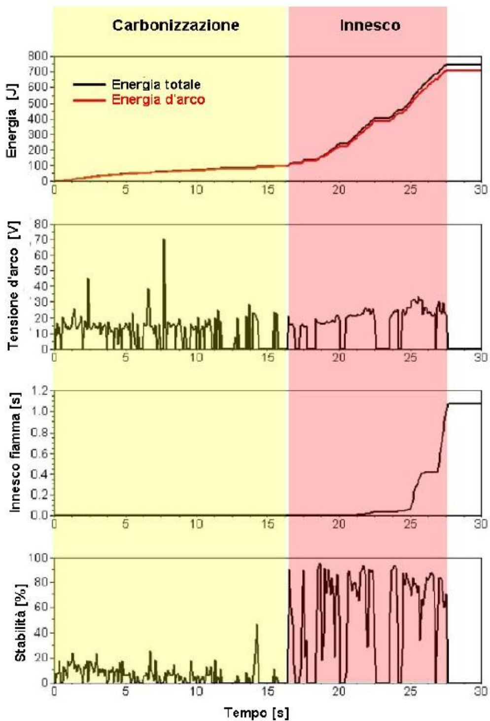
Figura 17: Simulazione di arco serie 5 A / 240 V
