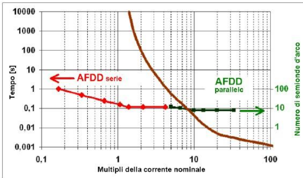
Figura 22: Protezione con fusibili classe gL (In=16A)
