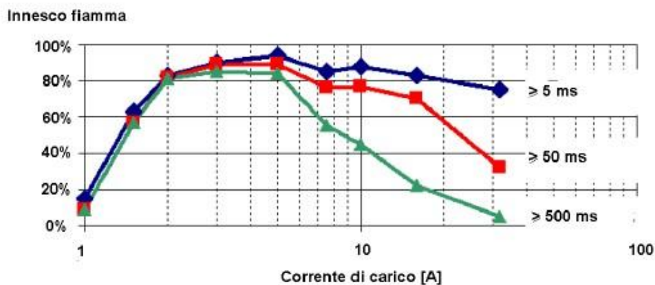
Figura 19: Tempi d'innesco in funzione della corrente di carico.
