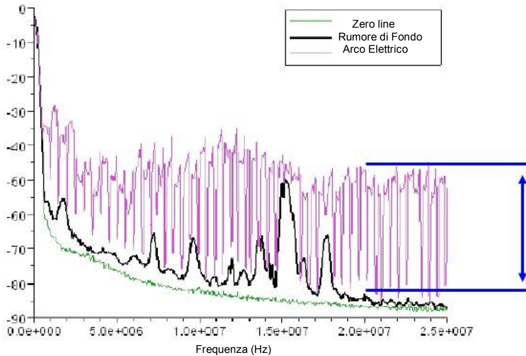
Figura 28: Analisi ad alta frequenza, rumore di fondo e rumore d'arco.
