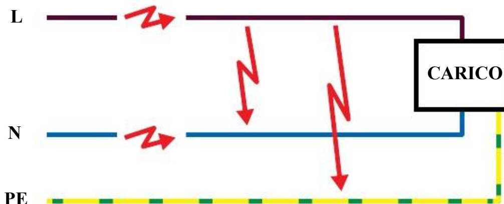
Figura 11: Tipologie di guasti da arco elettrico
