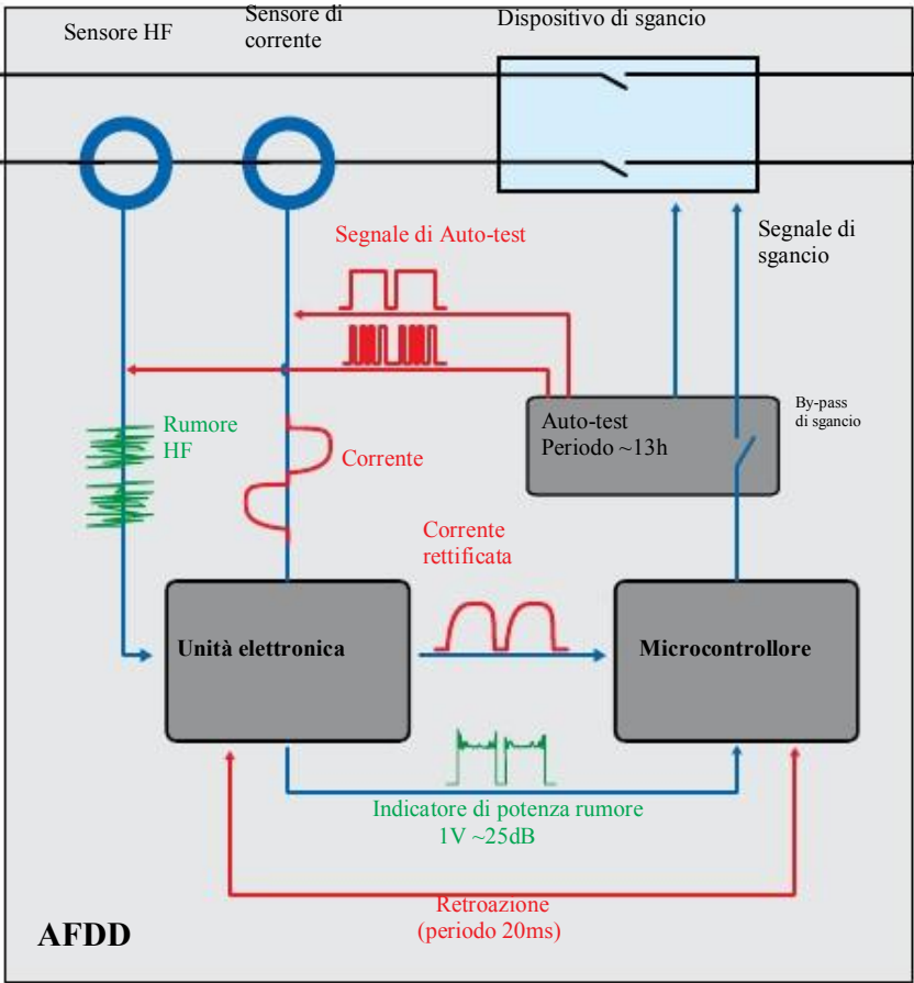
Figura 31: Diagramma relativo alla funzione interna di autotest
