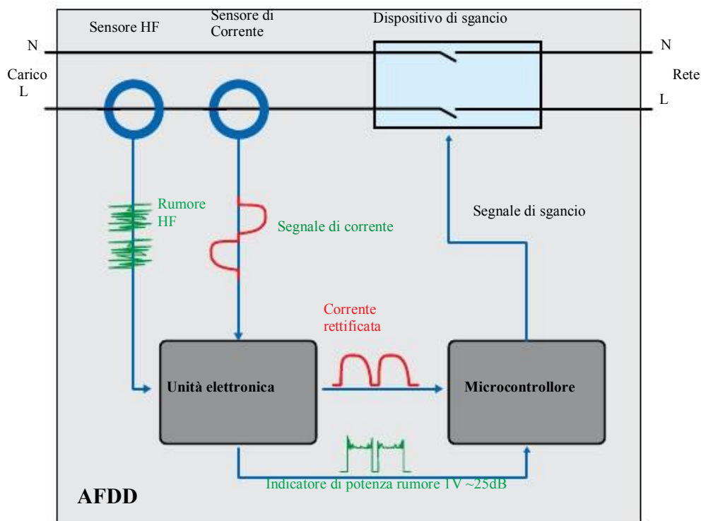
Figura 23: Struttura interna del AFD 5SM6
