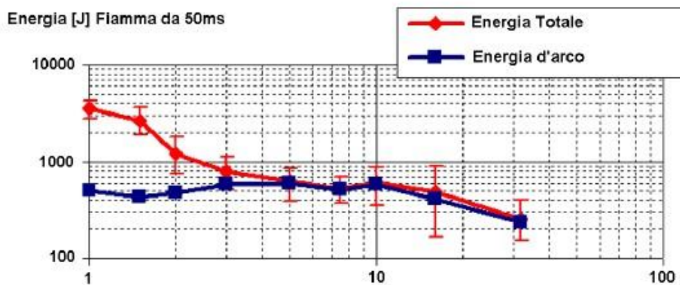
Figura 18: Energia d'innesco in funzione della corrente di carico.
