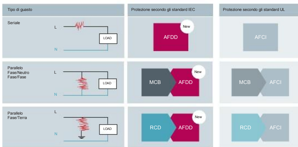
Figura 12: Tipologie di guasto e dispositivi idonei alla protezione.
