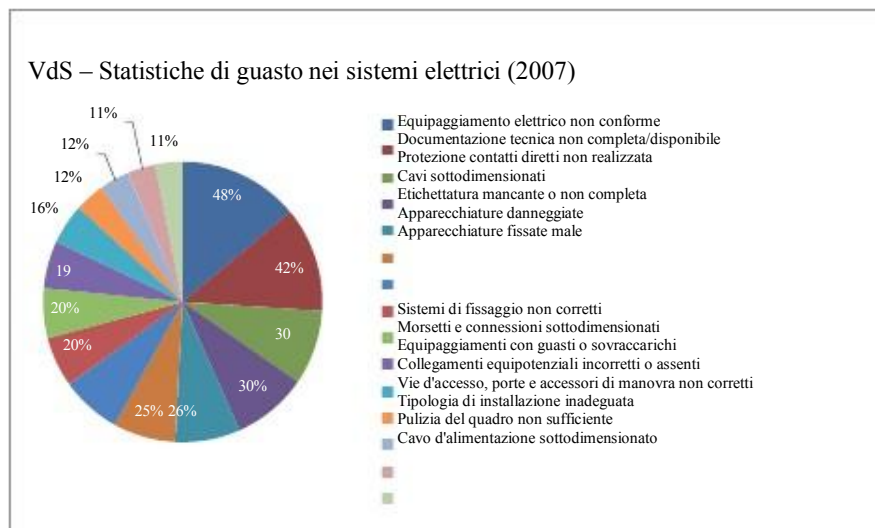
Figura 2: Statistiche di guasto nei sistemi elettrici (2007)
