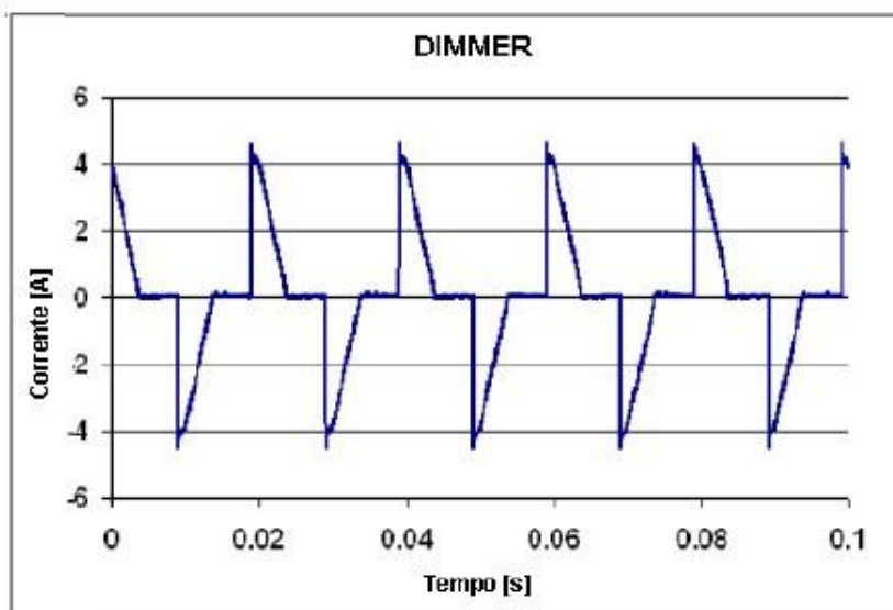
Figura 26: Esempio di carico elettrico con assorbimenti in alta frequenza
