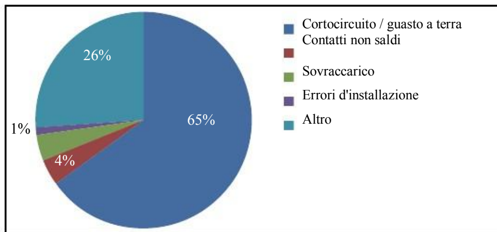
Figura 4: Finlandia: Statistiche d'incendio 2006 su 1.860 casi.
