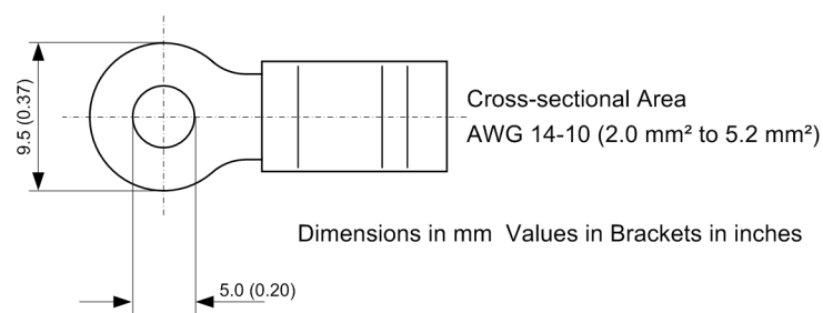
Figure 3-5 Ring lug
