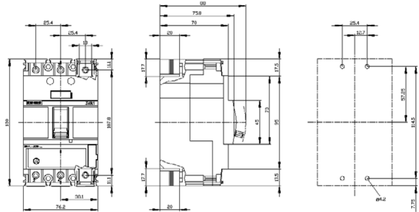
> 3VA10 / 3VA11, 3 Polos
