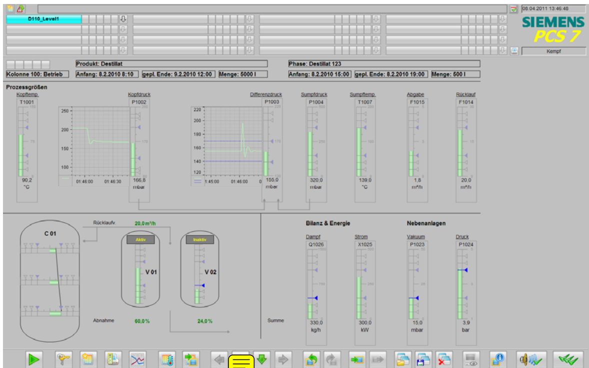
Fig. 2: Overview diagram of the column BILD DEUTSCH
