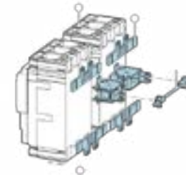
Enclavamiento posterior
