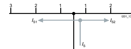
Conexión central 100/130 Amp.
