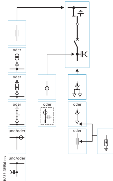
Dreistellungs-Trennschalter
