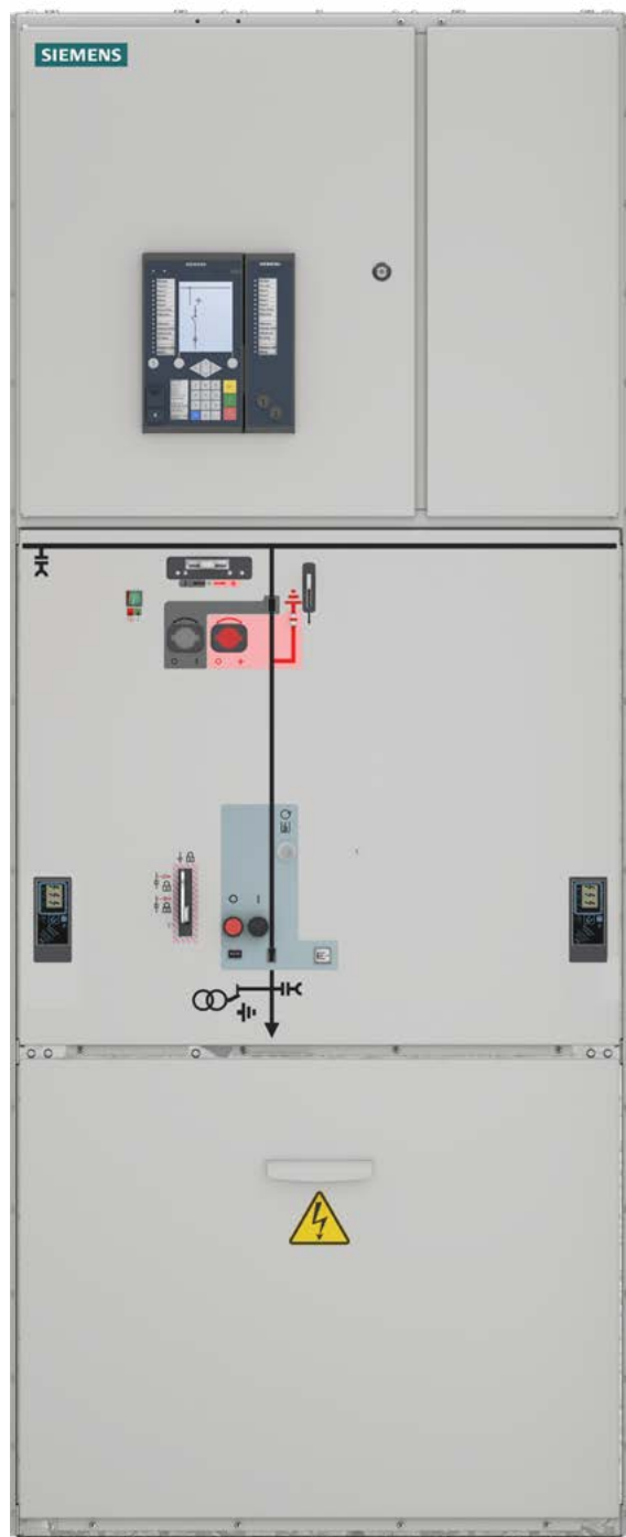
Leistungsschalterfeld 900 mm
