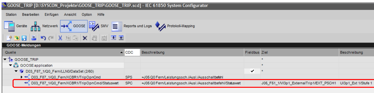
Bild 4: IEC 61850 Systemkonfigurator
